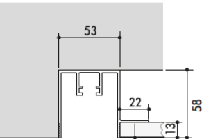
profilo ad incasso 1 via per parete e controsoffitto
