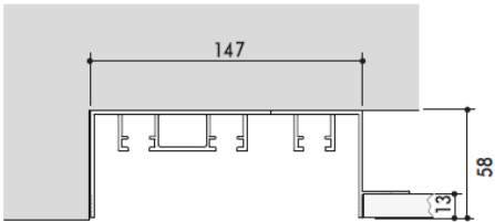
profilo ad incasso 3 vie per parete e controsoffitto
