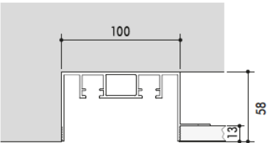
profilo ad incasso 2 vie per parete e controsoffitto
